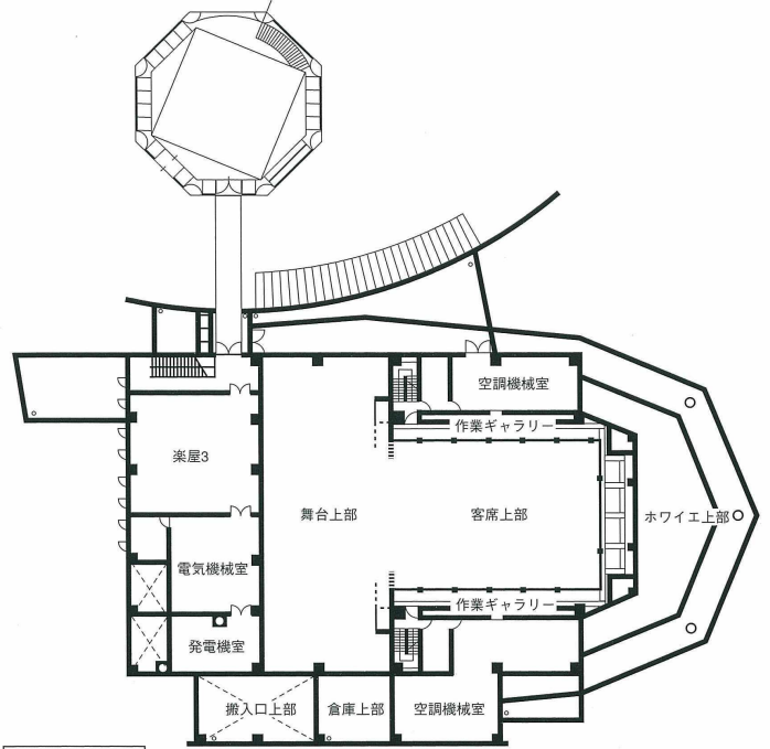
2階平面
