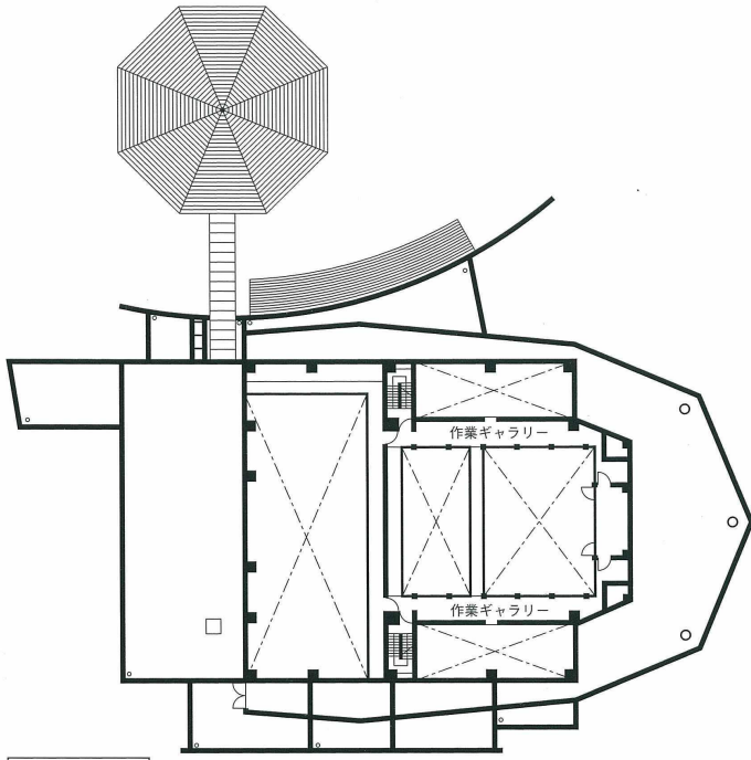
3階平面
